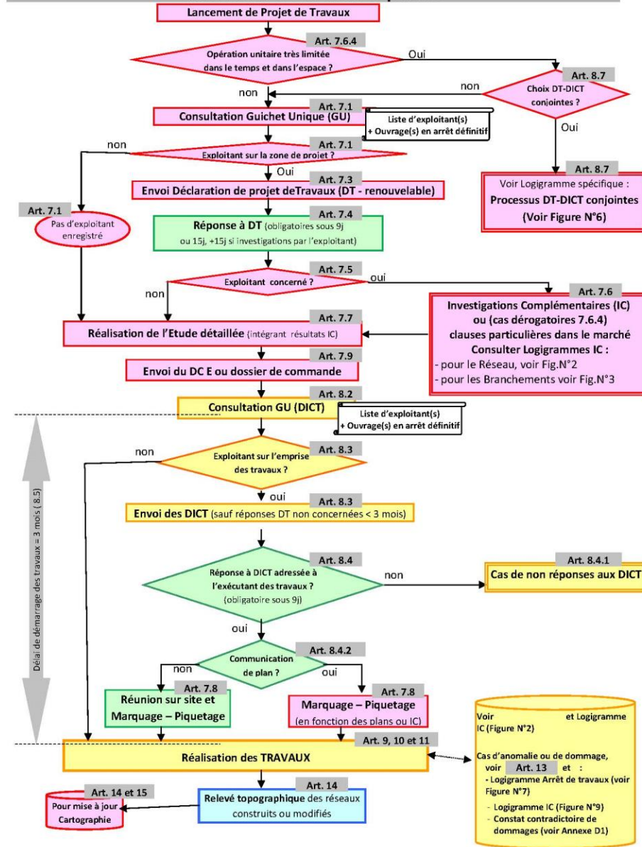
Figure N°1 : Logigramme général
